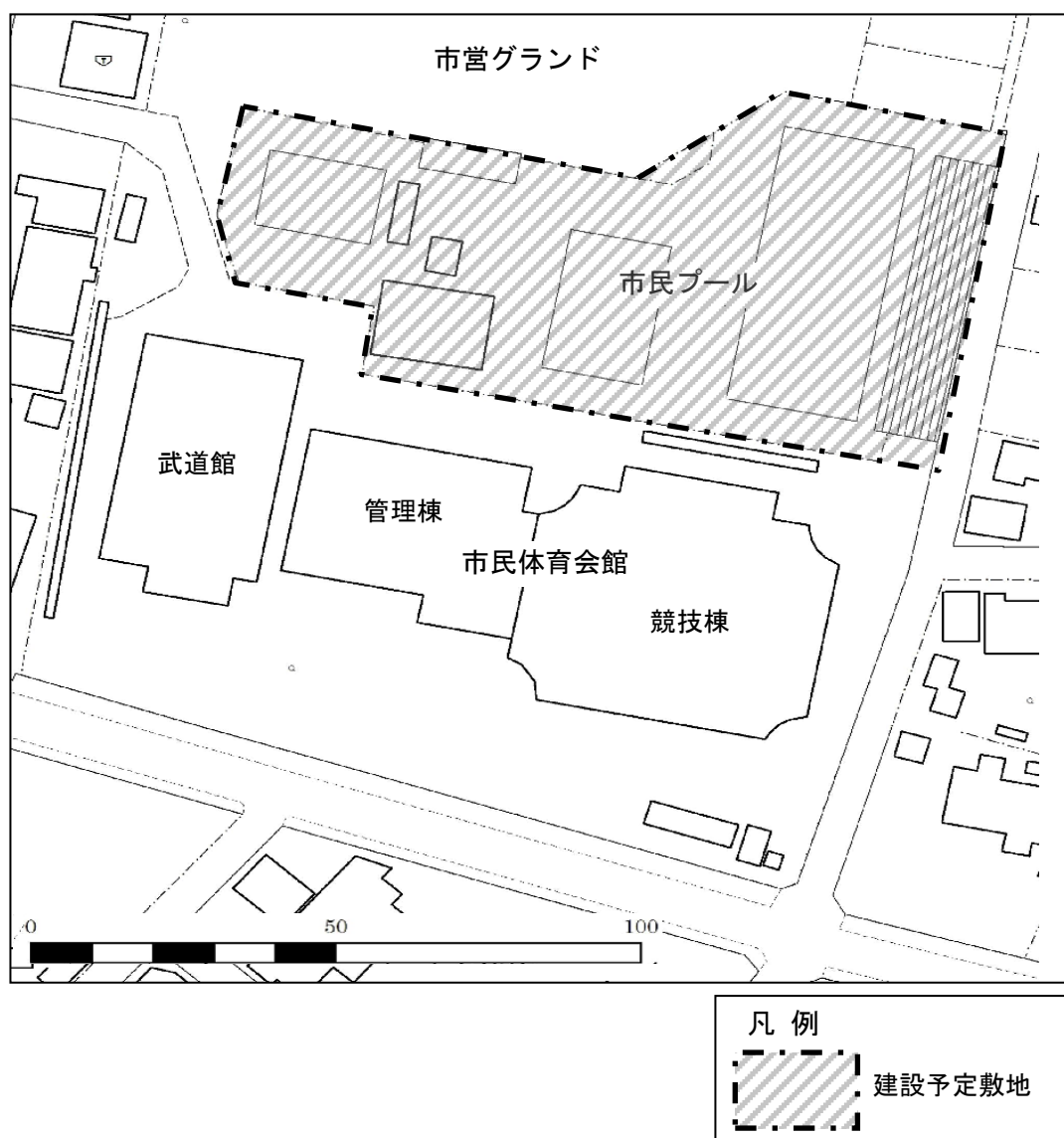
図表4-1 建設予定の敷地位置図
