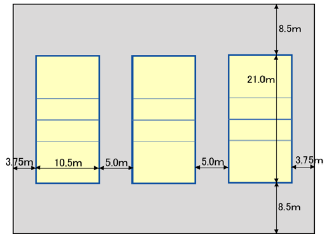
b : バレーボール9人制3面 (国内公式規格)
