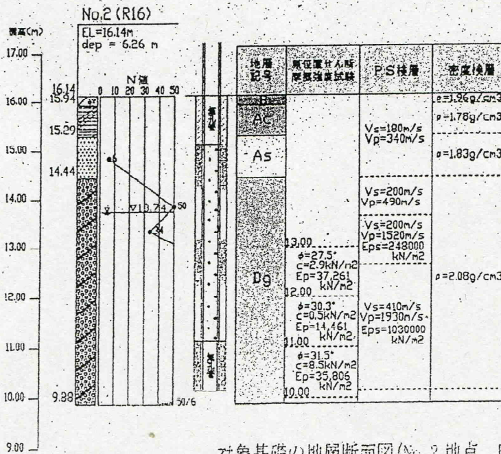
対象基礎の地層断面図(No. 2 地点, R16)
