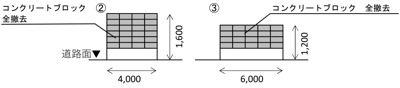
西側立面図
