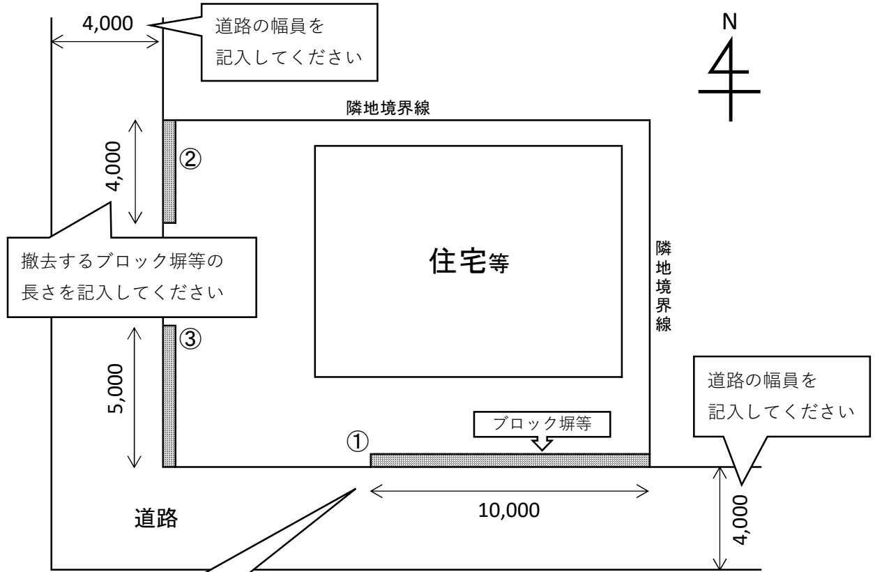
配置図
