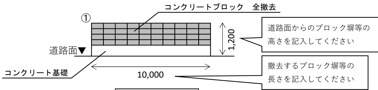
南側立面図
